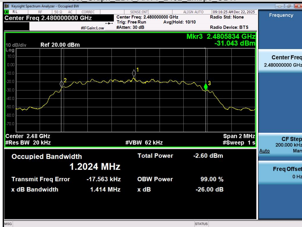
Test_Graph_EDR_ANT1_2480_2Mbps_OBW
