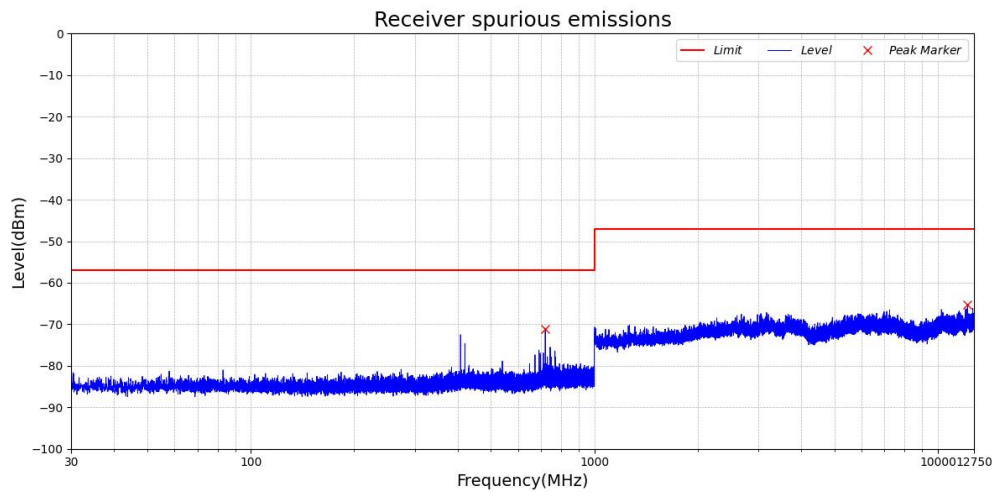
Test_Graph_ANT1_2402_1Mbps_RX
