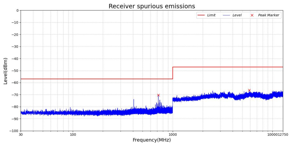
Test_Graph_ANT1_2480_1Mbps_RX
